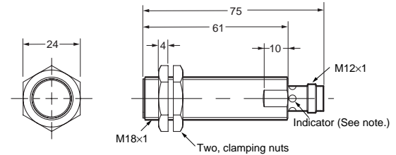
E2AU-M18LS08-M1-□□
